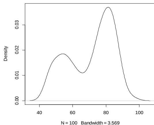
Fig. 4 bcv –Default Bandwidth
