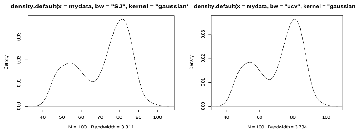
Fig. 2 SJ –Default Bandwidth
